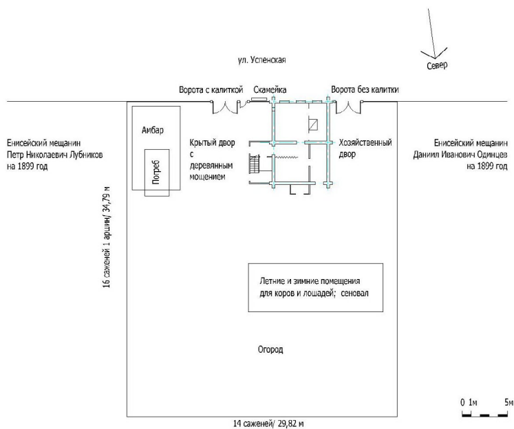
Ил. 5. План усадьбы Бурдаковых. Схема С.Ю. Слободчикова Fig. 5. A plan of Burdakov's farmstead. Scheme by S.Y. Slobodchikov
