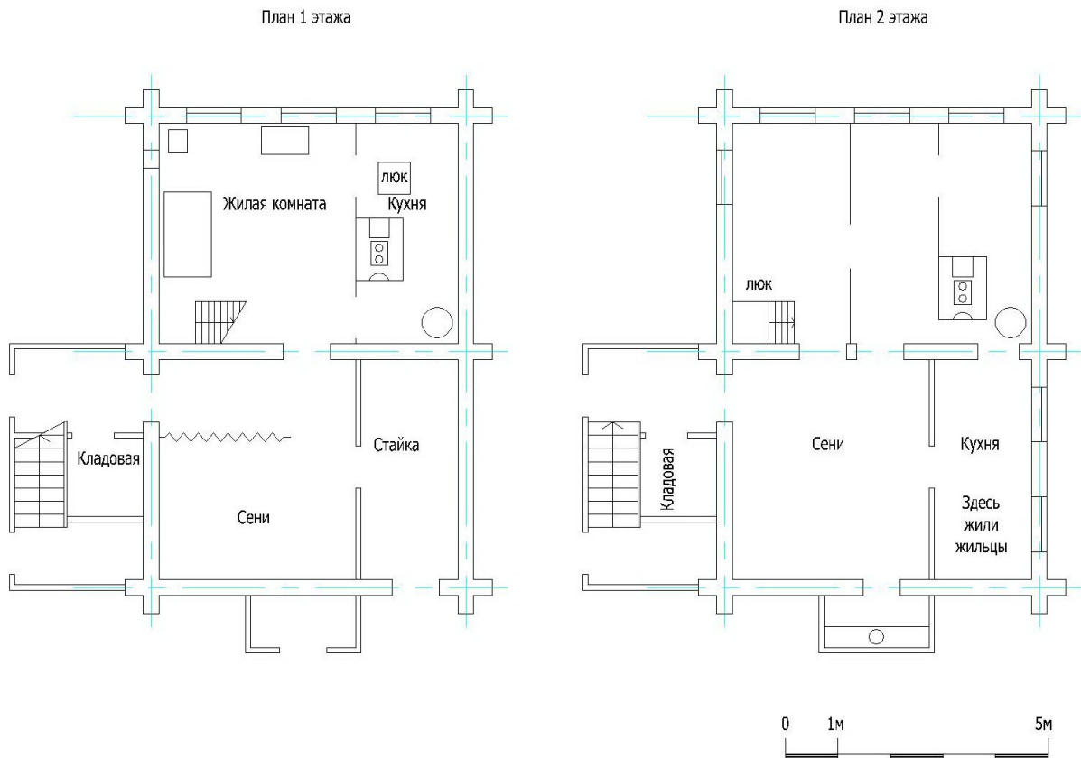
Ил. 4. План дома Бурдаковых. Схема С.Ю. Слободчикова Fig. 4. A plan of Burdakov's house. Scheme by S.Y. Slobodchikov
